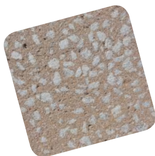
LIMONITE
