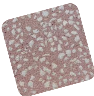
SCHISTE
