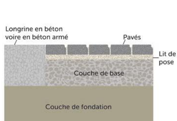
Figure 29 - Exemple de blocage des rives au moyen d'une longrine en béton.
