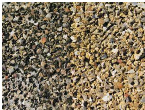
Photo 98 - Aspect du béton drainant avant nettoyage (partie gauche) et après nettoyage (partie droite).
